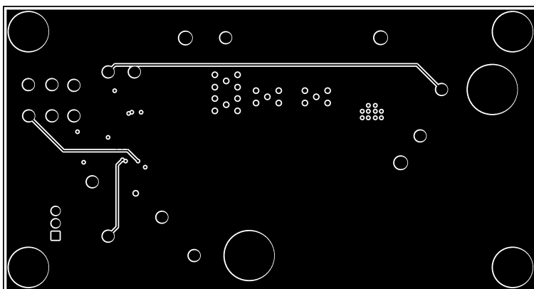
Figure 4-6. Layer 3
