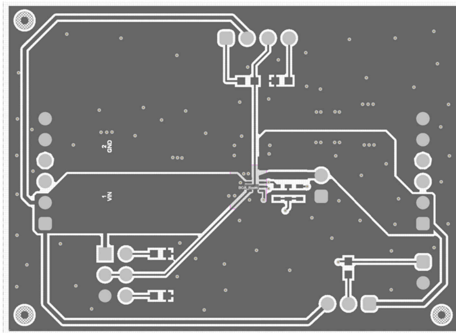
Figure 6-2. Top Layer
