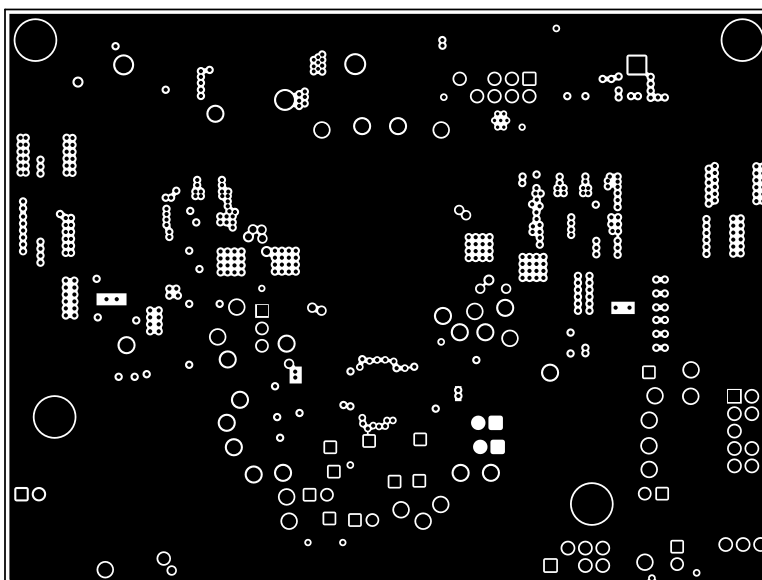
Figure 4-6. Layer 2 -GND
