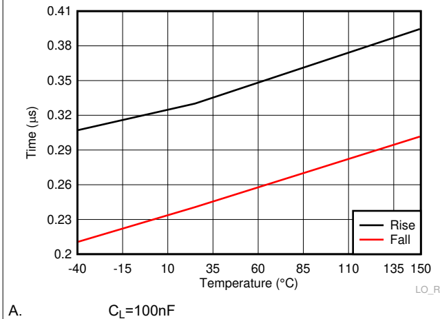
Figure 6-21. LO Rise andamp; Fall Time
