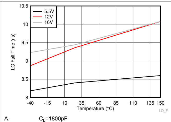
Figure 6-18. LO Fall Time
