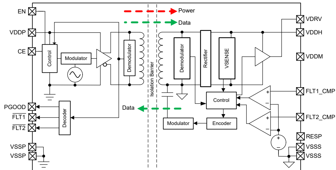
Figure 8-2. TPSI311x-Q1, TPSI311xL-Q1
