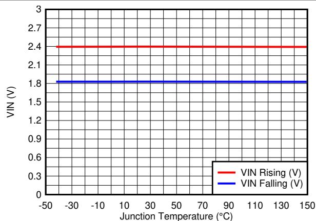
Figure 5-7. VIN UVLO
