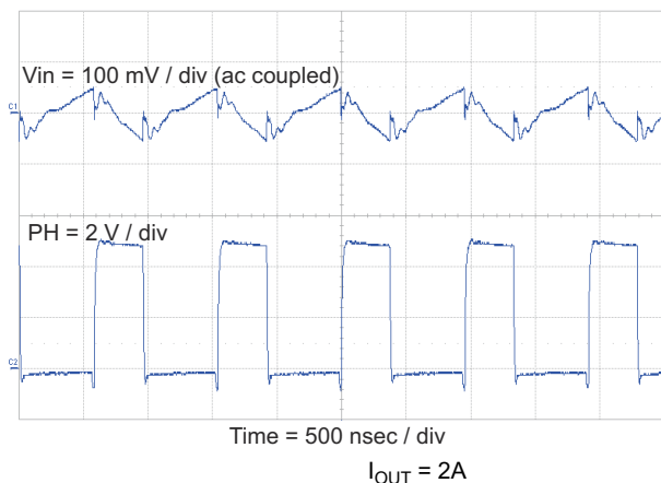
Figure 8-8. Input Ripple
