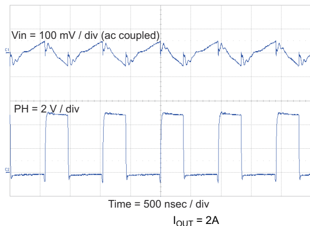
Figure 8-8. Input Ripple
