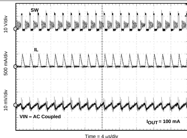
Figure 45. Input Ripple DCM
