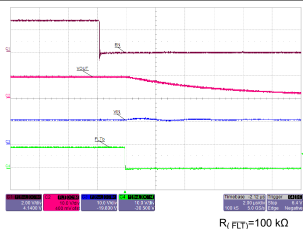
Figure 7-35. EN Turn OFF Delay : EN ↓ to Fault ↓
