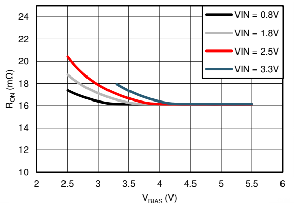
Figure 7-9. R_{ON} vs V_{BIAS}
