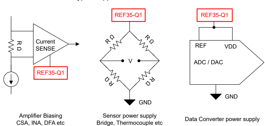
REF35-Q1 Use Case
