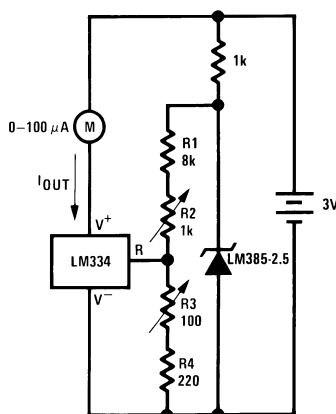
Figure 16. 0°C–100°C Thermometer
