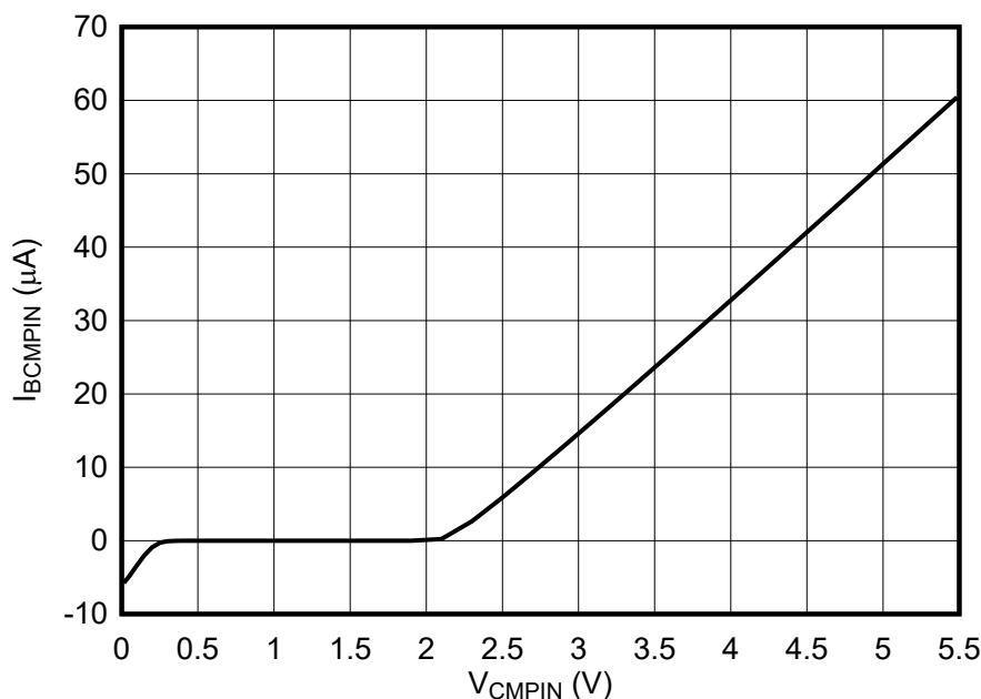
Figure 7-3. Comparator I_{BCMPIIN} vs V_{CMPIIN}
