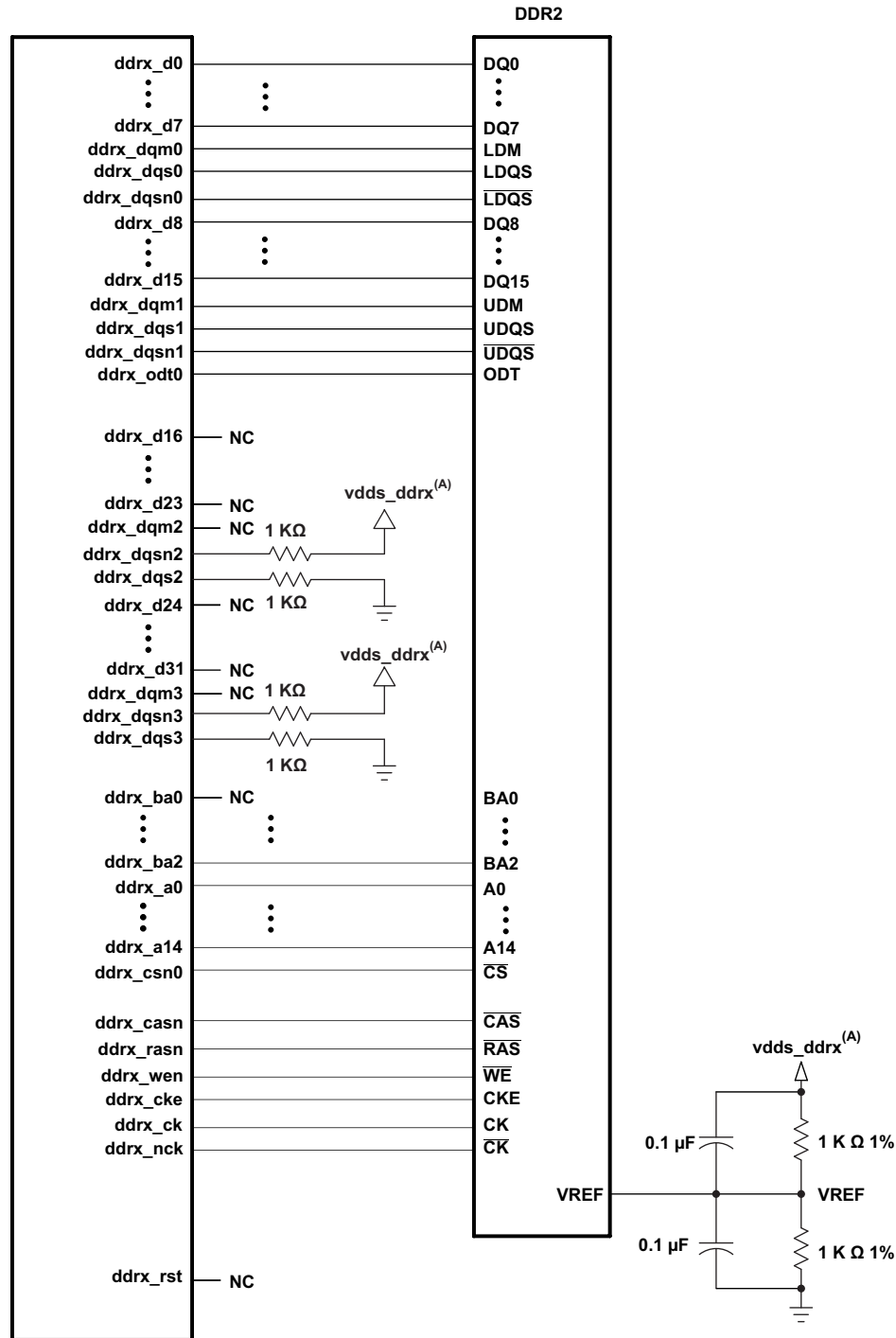
PCB_DDR2_2
