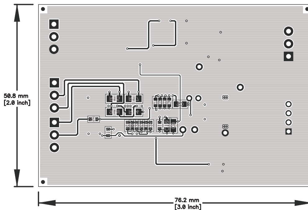
Figure 24. Bottom Layer
