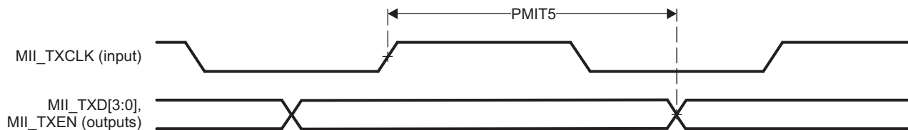
Figure 5-127. PRU-ICSS MII_TXD[3:0], MII_TXEN Timing
