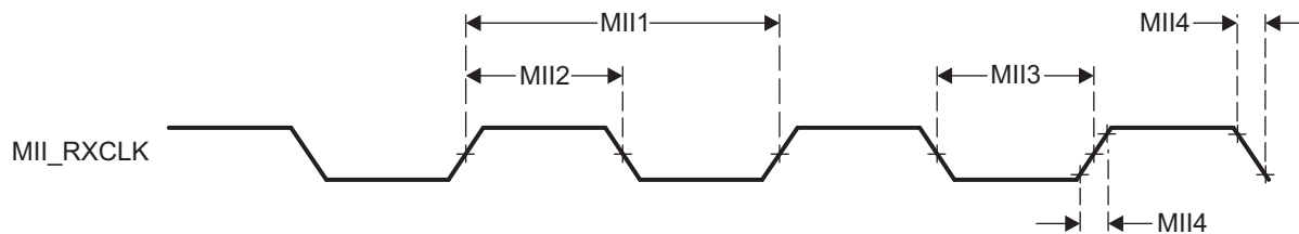
EMAC_MII_01
