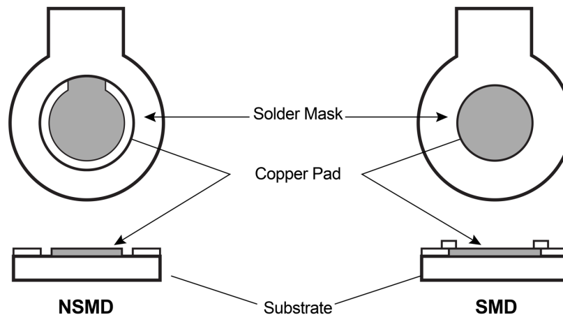
그림 6. NSMD 및 SMD PCB 랜드 패턴
