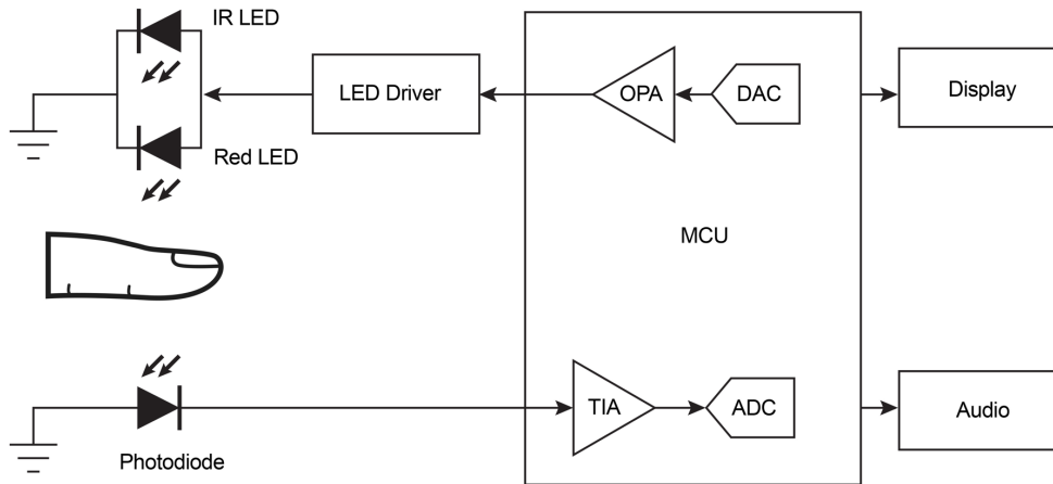
그림 4. 통합 부품을 사용한 펄스 옥시미터 설계
