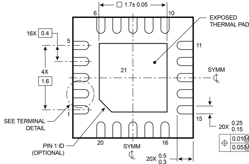
그림 1. 20핀 0.8mm QFN 패키지의 MSPM0C1104 그림
