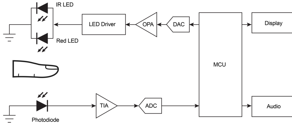
그림 3. 개별 아날로그 부품을 사용한 펄스 옥시미터 설계
