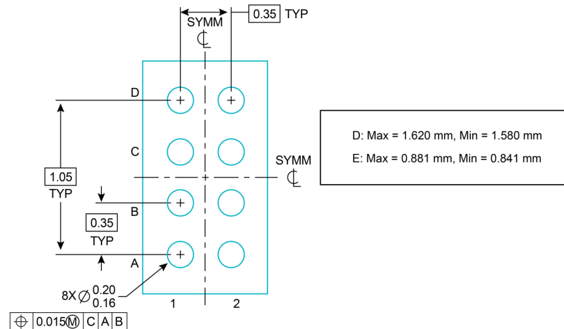
그림 2. MSPM0C1104 8볼 WCSP 패키지 그림(공칭 1.50 x 0.86mm, 두께 0.35mm)
