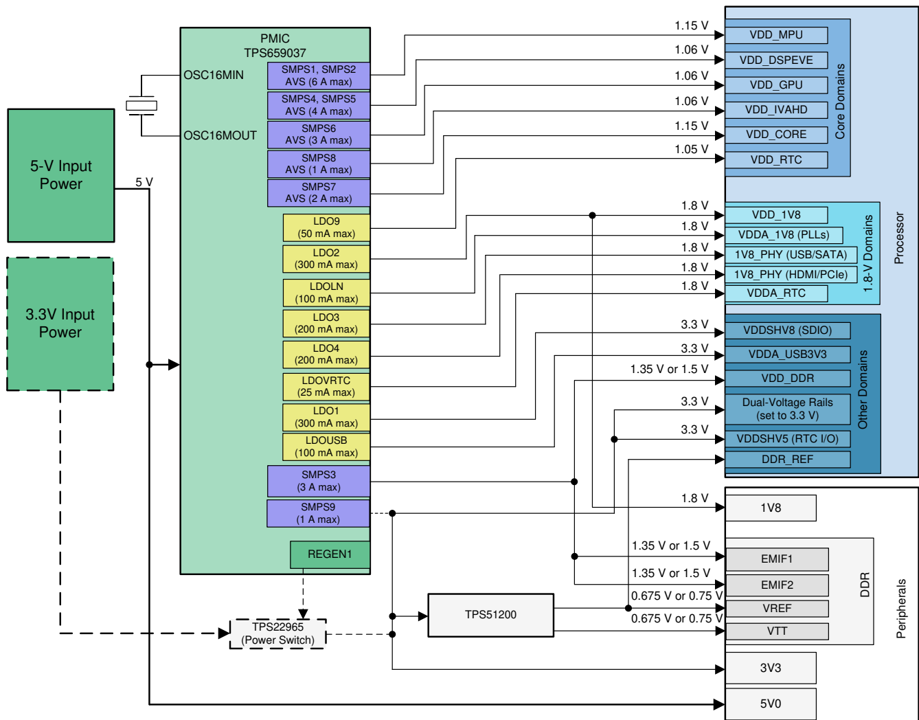
図 2-6. TPS6590379 PMIC から AM574x プロセッサへの接続
