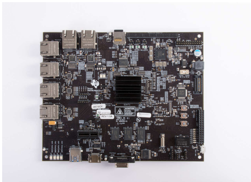
図 2-1. AM574x IDK EVM - 上面図
