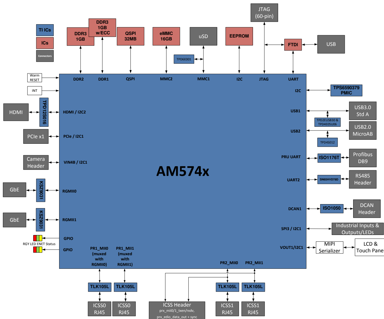
図 2-5. AM574x IDK EVM のブロック図
