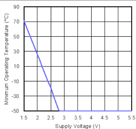
図 6-2. 最低動作温度と電源電圧との関係
