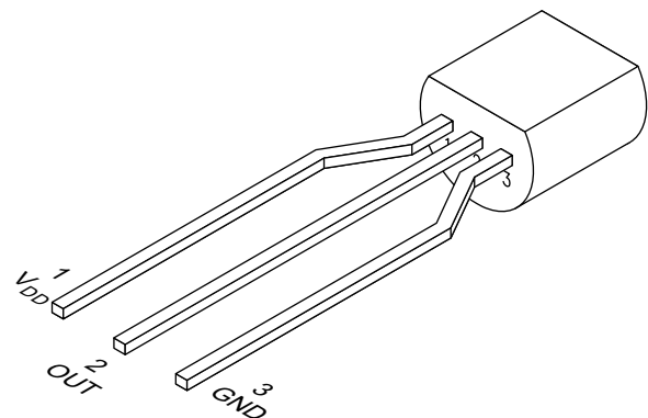
図 5-4. LPM パッケージ、3 ピン TO-92 (上面図)
