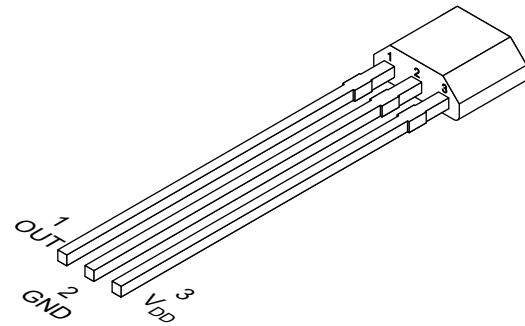
図 5-2. LPG パッケージ、3 ピン TO-92S (上面図)
