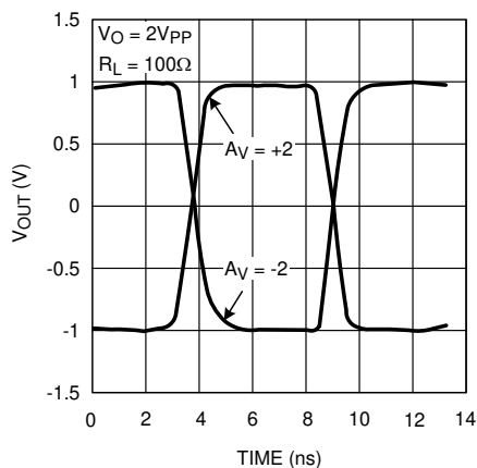
図 5-7. Step Response, 2Vpp
