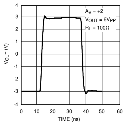
図 5-8. Step Response, 6Vpp
