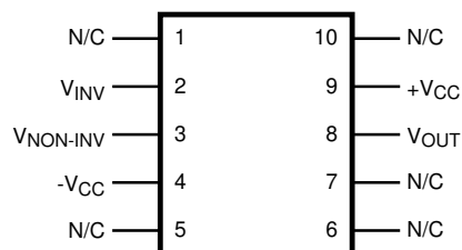
図 4-2. NAC Package, 10-Pin CLGA (Top View)
