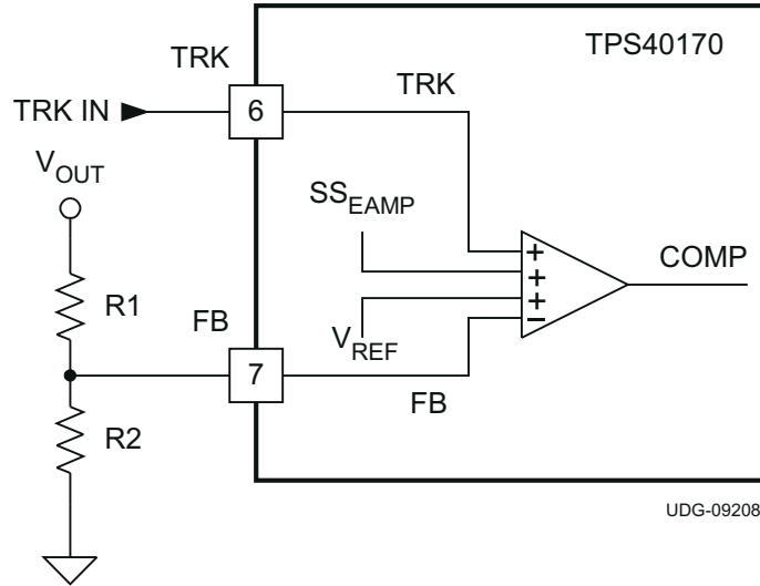
図 6-9. Tracking Functional Block
