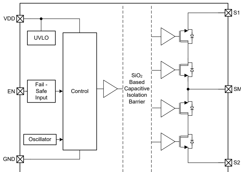
8-1. TPSI2140-Q1 Block Diagram
