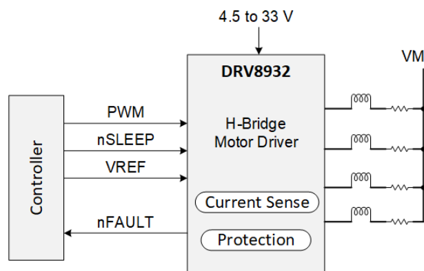
DRV8932 の概略回路図
