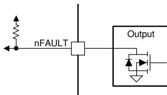
図 7-13. nFAULT ピン
