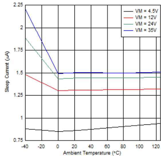
図 6-2. スリープ電流と温度との関係
