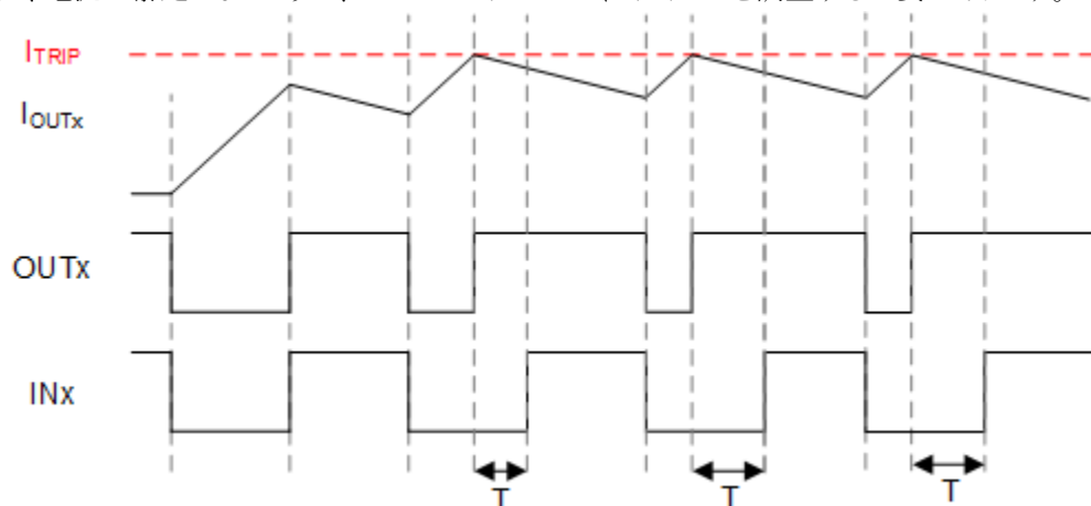
図 7-6. VM に接続された誘導性負荷、サイクル単位の制御、T は DRV8932 の T_{OFF} よりも小さい必要があります。
