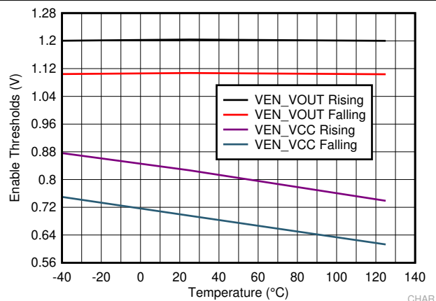
FIG 6-8. Enable Thresholds
