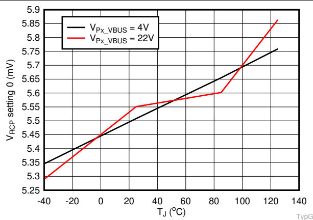
图 6-3. V RCP vs. Temperature
