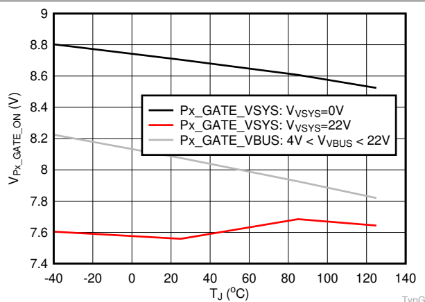
图 6-5. V Px_GATE_ON vs. Temperature
