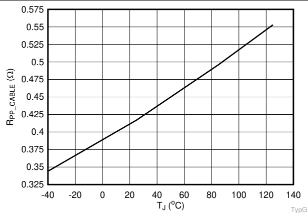
图 6-2. PP_CABLEx Rdson vs. Temperature
