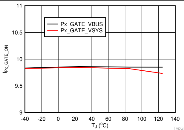
图 6-6. I Px_GATE_ON vs. Temperature
