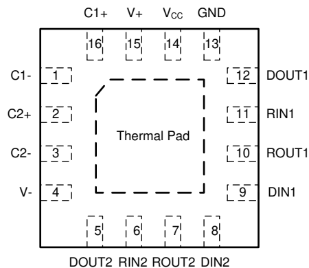
図 4-2. RGT package, 16 Pin VQFN, Top View
