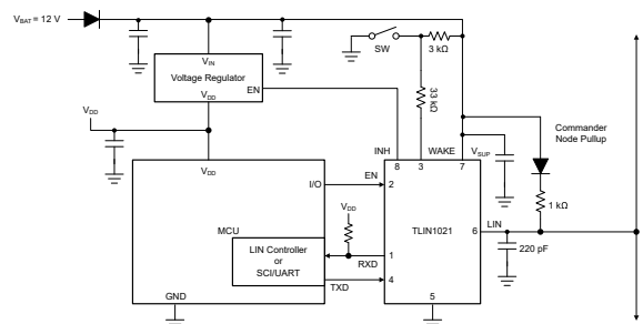
コマンド・ノードの概略回路図
