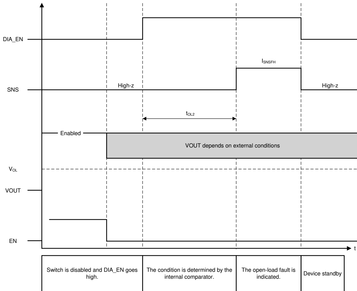
图 11. Open Load
