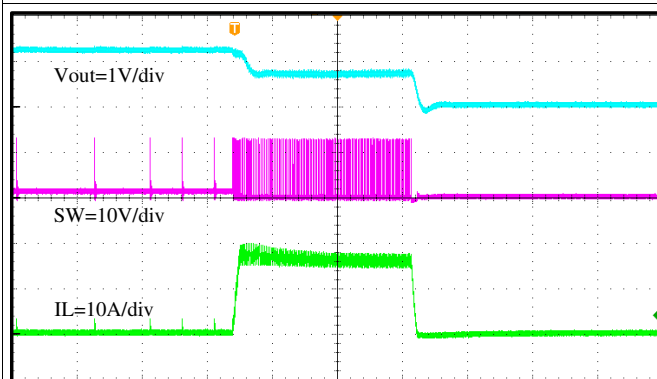
图 31. Transient Response
