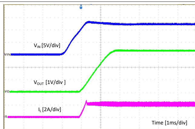
FIG 15. DCM Mode
