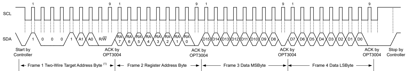
图 8-2. I 2 C Write Example
