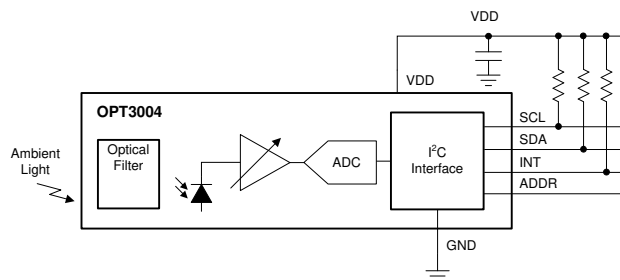
ブロック図
