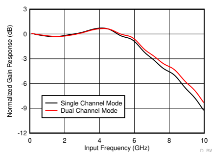
ADC12DJ3200QML-SP で測定された入力帯域幅
