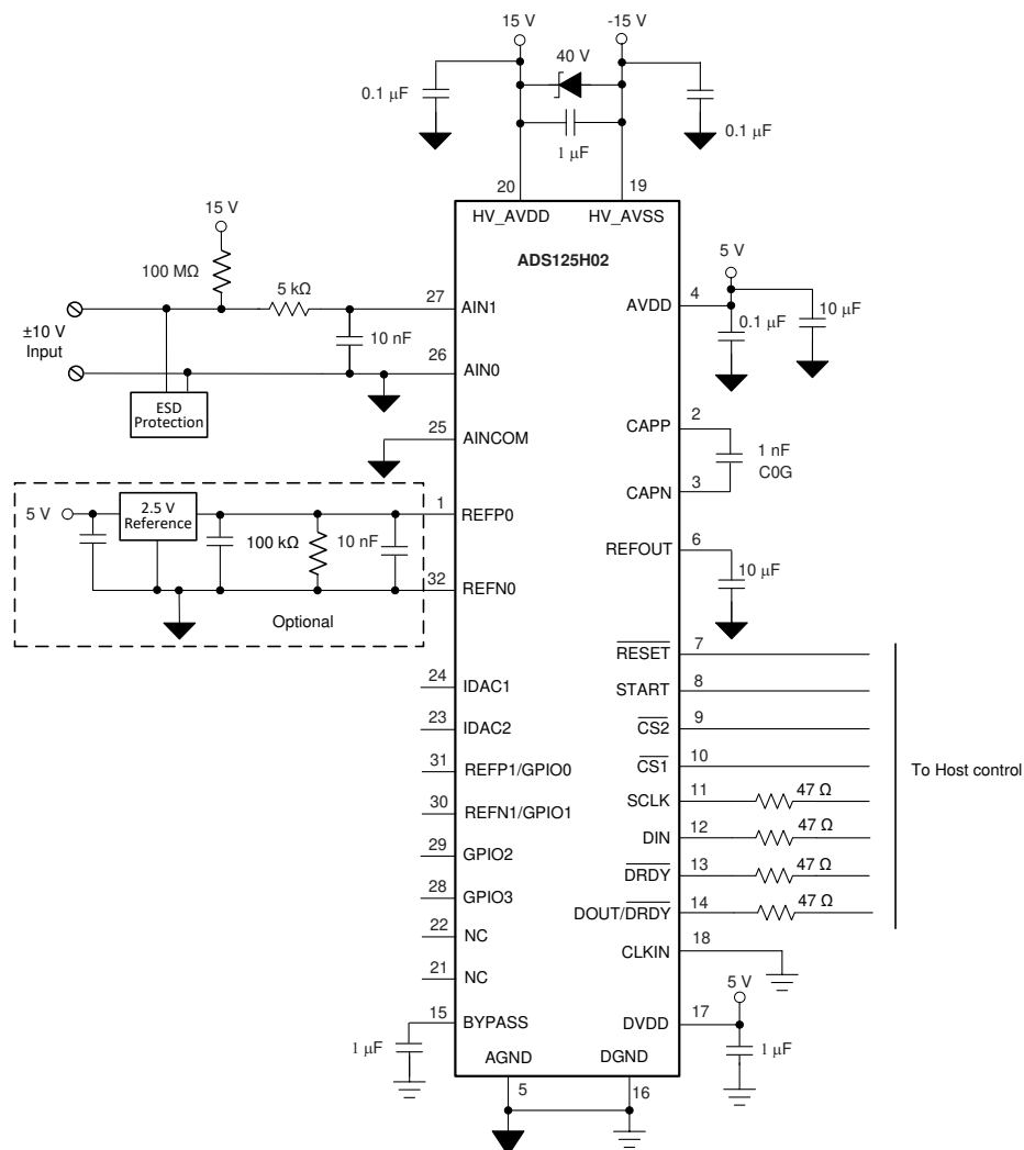
图 98. \pm 10\text{-V} Analog Input PLC Module
