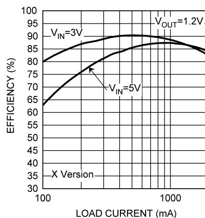
図 5-4. Efficiency vs Load
