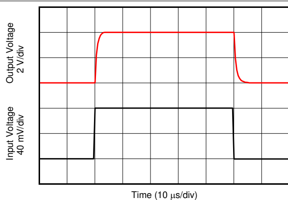
80mV PP の入力ステップ 図 6-31. ステップ応答
