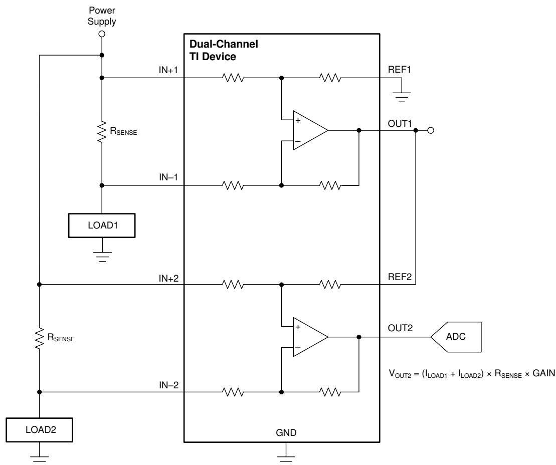
図 8-3. 複数の電流の加算
