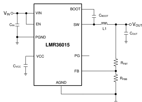
概略回路図
