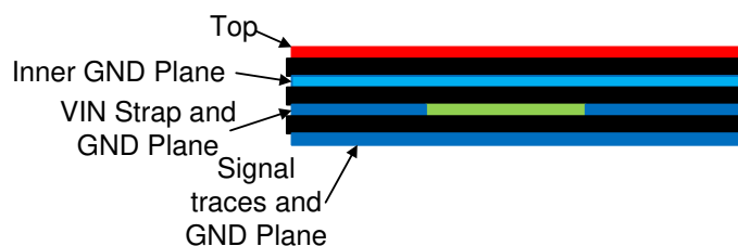
✎ 12-2. Example Layout
