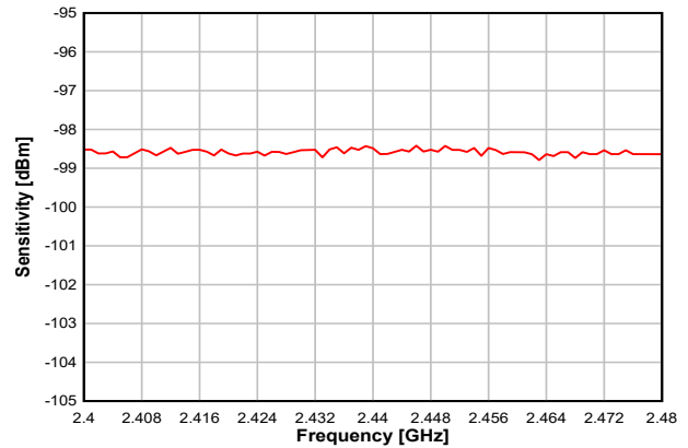
図 8-11. Sensitivity vs. Frequency (IEEE 802.15.4-2006, 250 kbps, OQPSK DSSS 1:8, 2.44 GHz)
