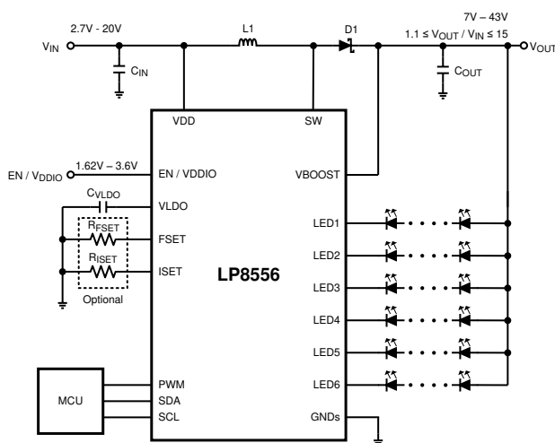
概略回路図
