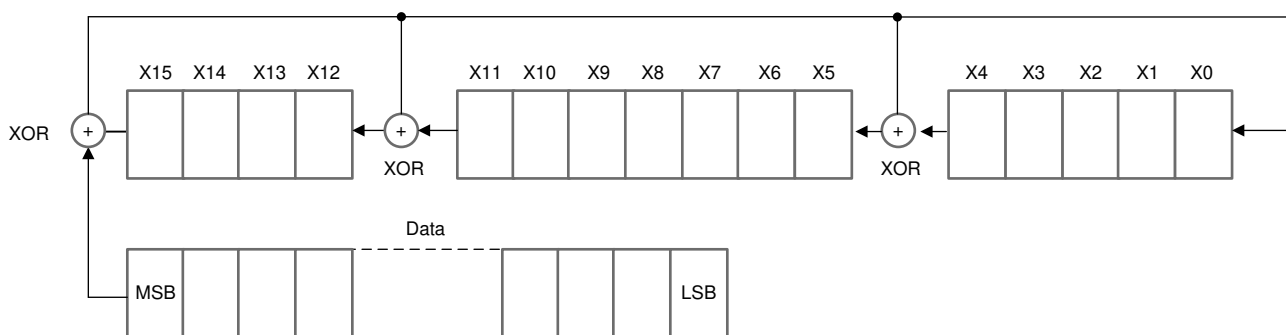
图 8-10. CCITT-16 CRC Module Block Diagram
