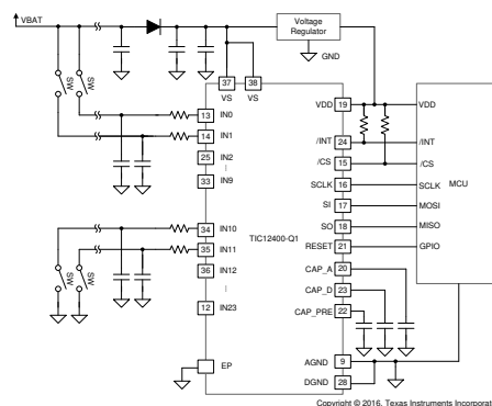
概略回路図
