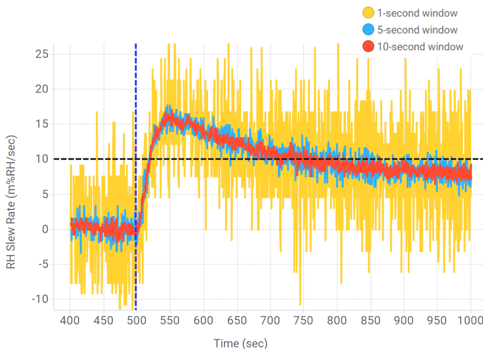
図 5-3. テスト 2 (22°C、45%RH、0.07mL 水):さまざまなタイム ウィンドウにわたって計算された RH スルー レート
