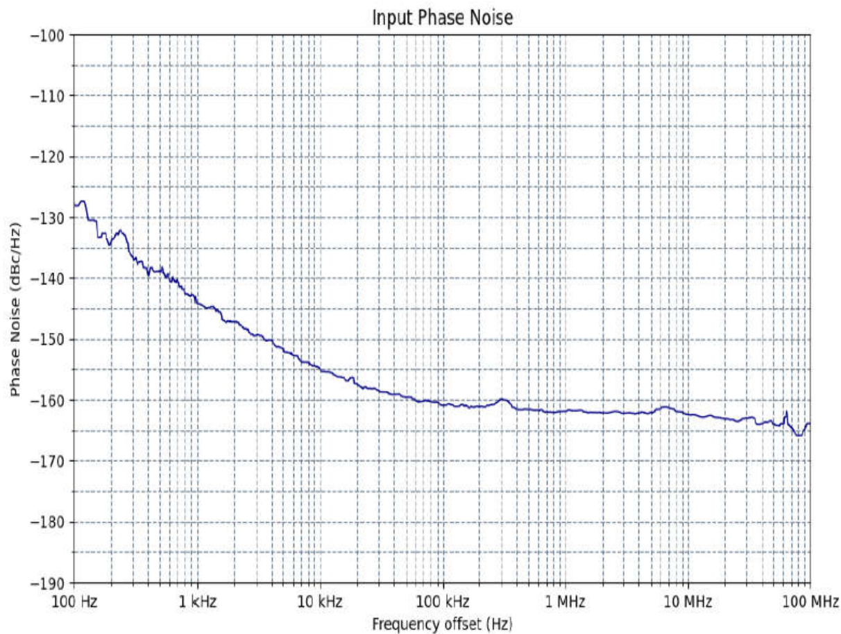
図 5-1. LMK00338 から LMK00338 デバイスへの 100MHz 基準入力信号が 3.5V/ns、ピークツーピーク スイング = 1.6Vpp であることによる出力位相ノイズ曲線
