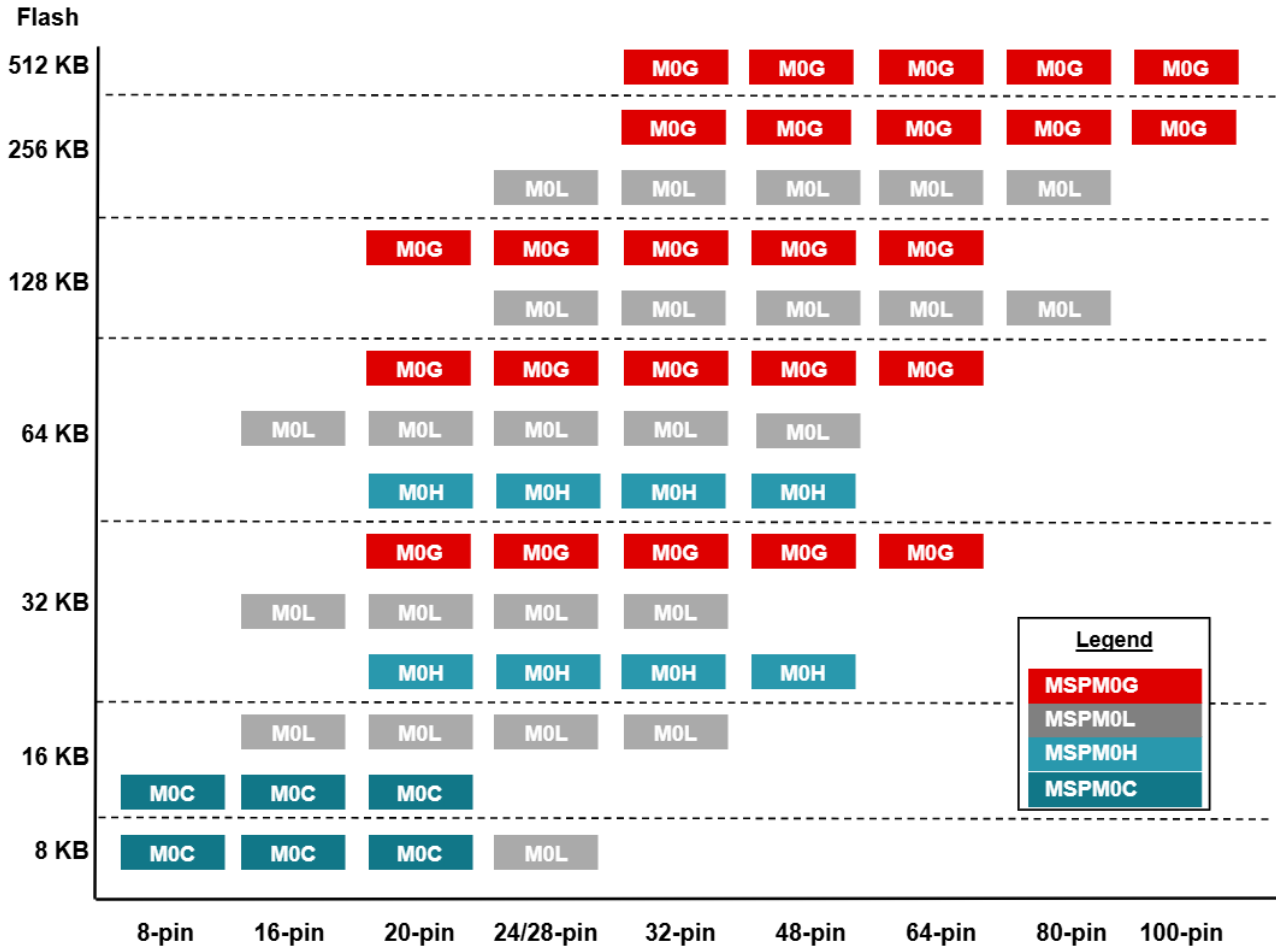
図 1-1. MSPM0 の製品ラインアップ
