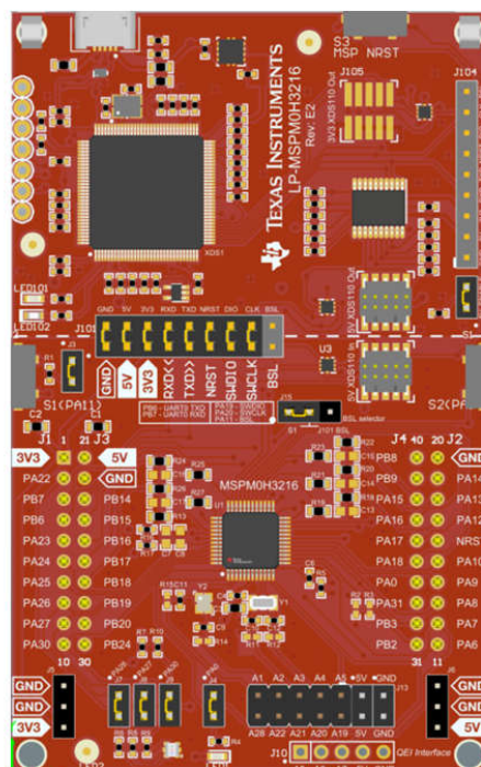
図 2-9. MSPM0Hxx LaunchPad キット
