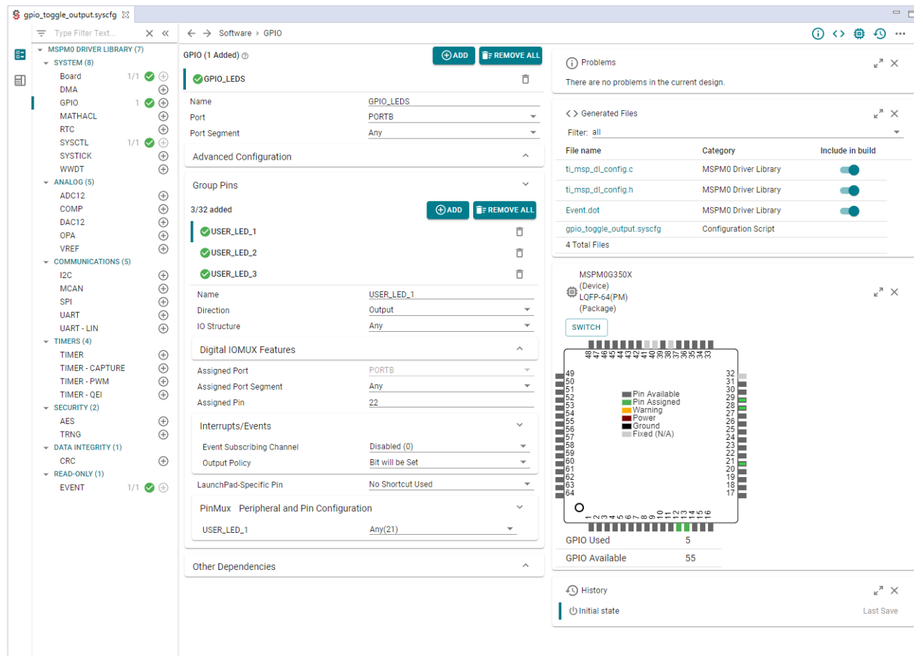
図 2-1. MSPM0 SysConfig の例
