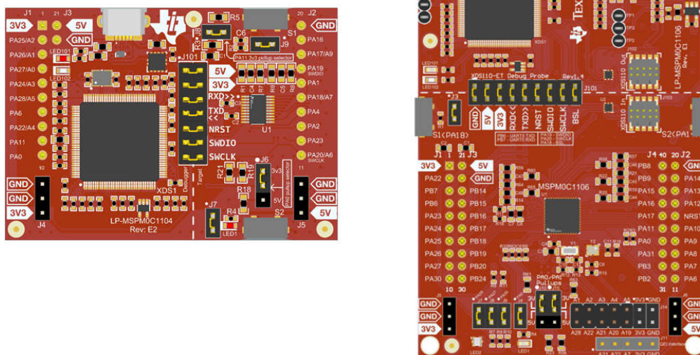
図 2-8. MSPM0Cxx LaunchPad キット
