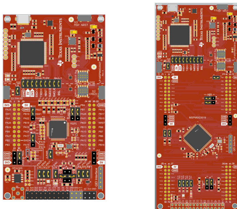
図 2-6. MSPM0Gxx LaunchPad キット
