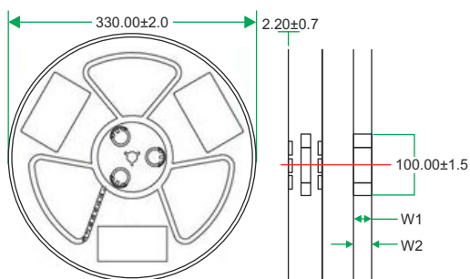
図 12-3. リール仕様
