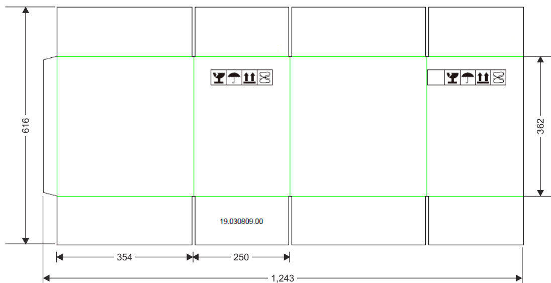
図 12-5. 梱包箱
