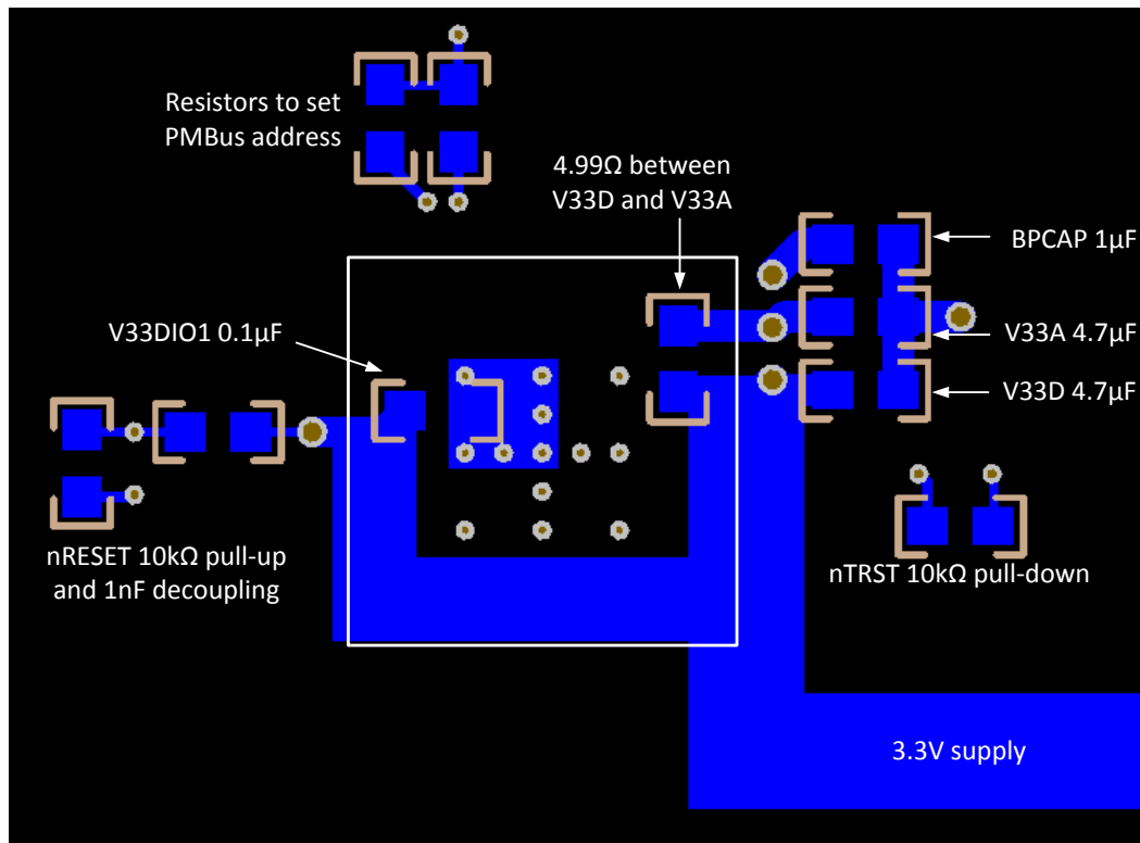
图 36. Example Layout – PCB Bottom Layer
