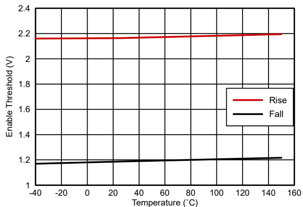
图 5-12. Enable Threshold
