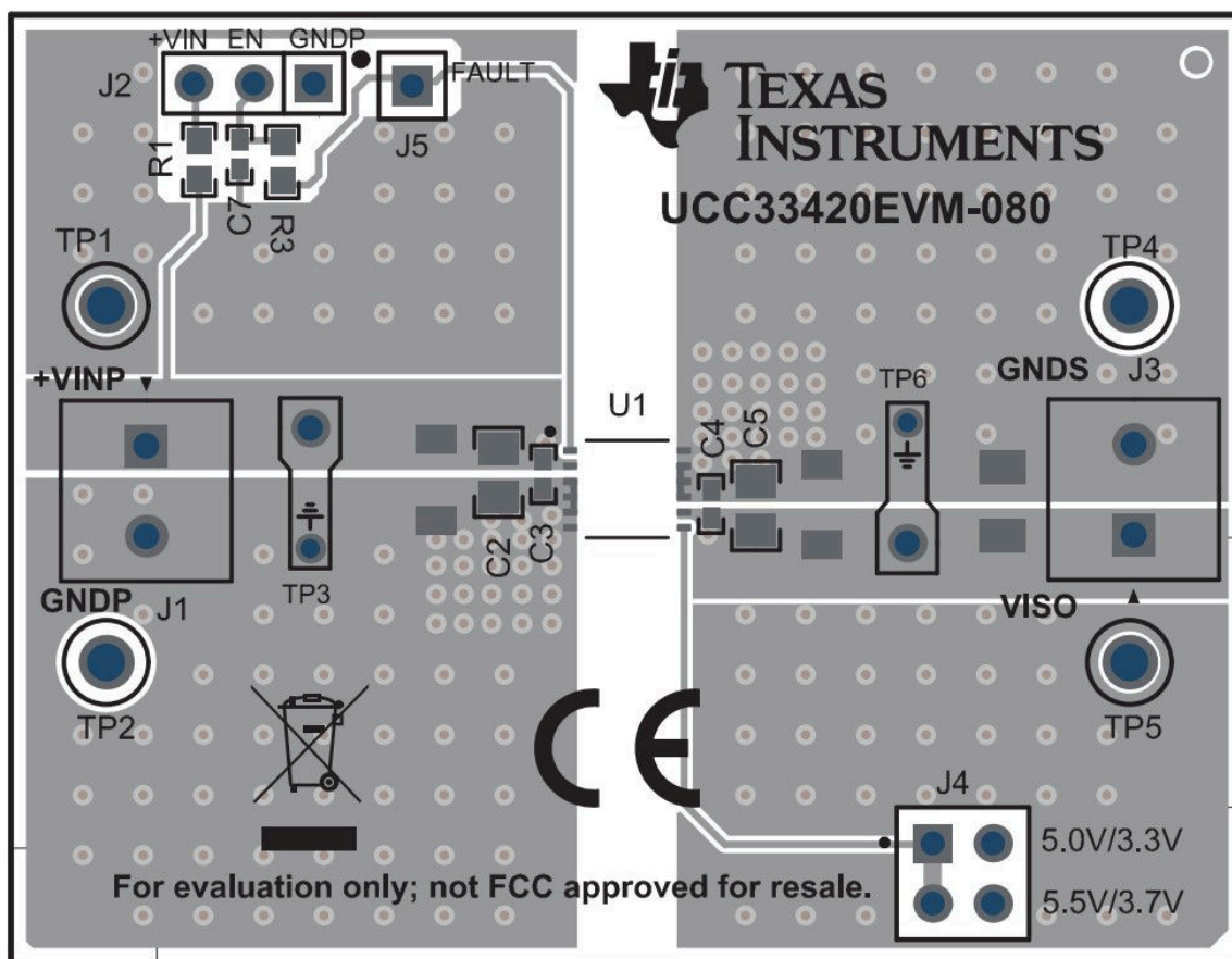
図 7-2. Layout Example
