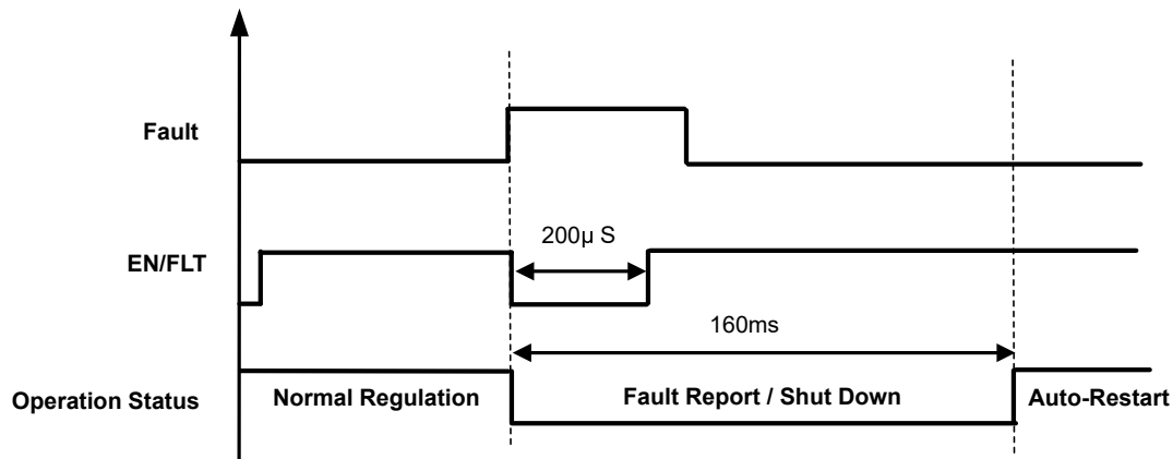
図 7-7. Auto-Restart Operation
