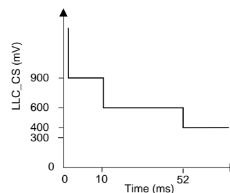
LLC 段の過電流保護プロファイル
