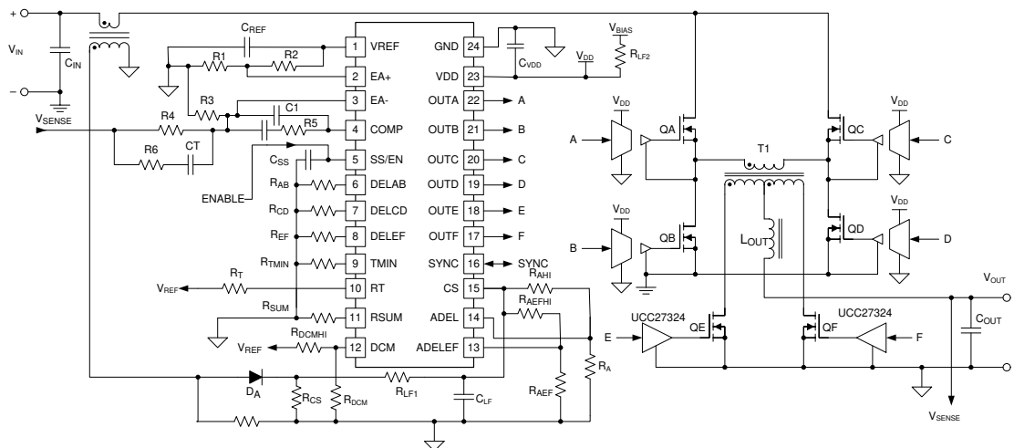
アプリケーション概略図
