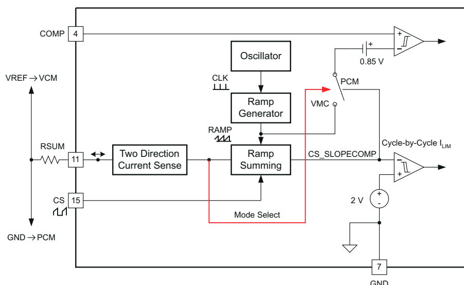
图 6-9. 斜坡补偿电路的操作逻辑
